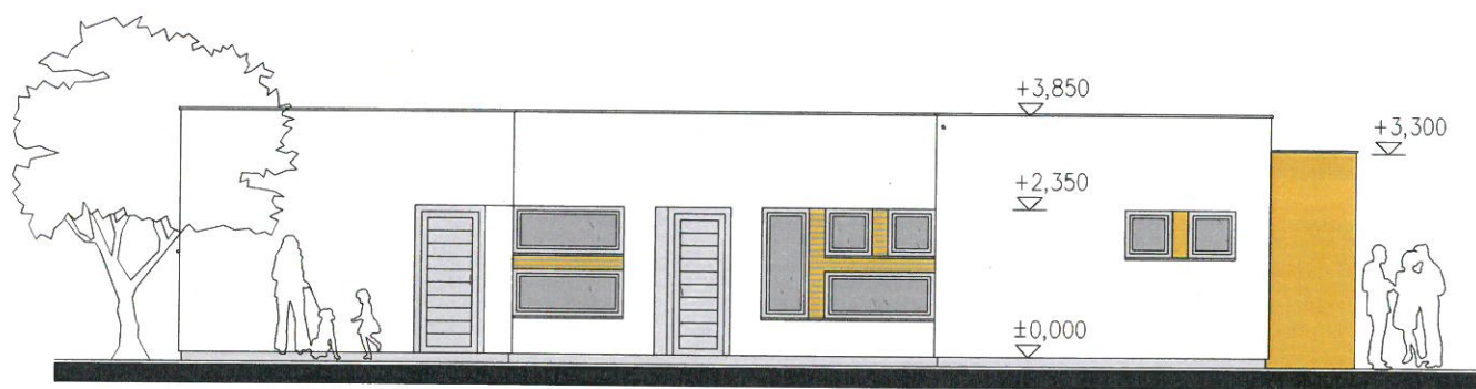
POHĽAD SEVEROVÝCHODNÝ
