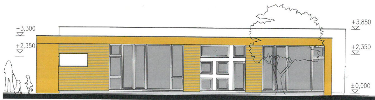
POHĽAD JUHOZÁPADNÝ
