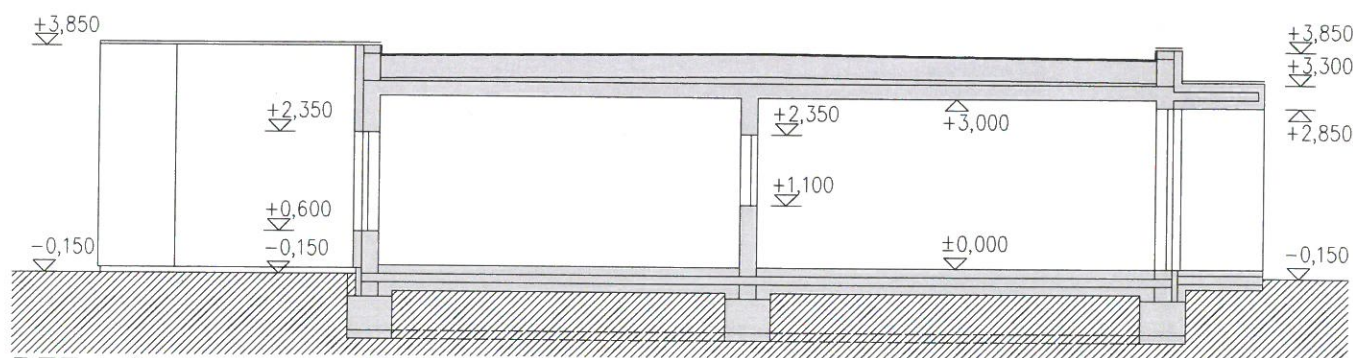
REZ A-A'
